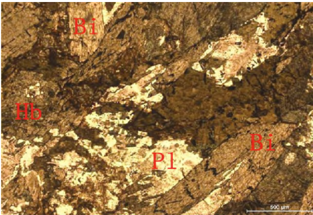
图3 JC12-1薄片单偏光5×,斜长角闪岩(左),JC113薄片正交偏光5×,混合花岗岩(右)
