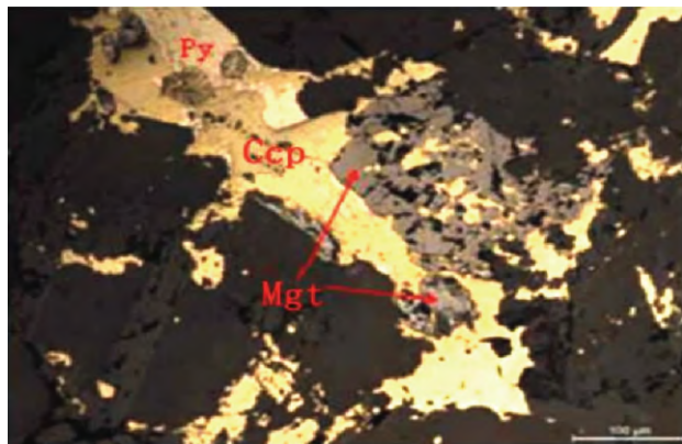
图11 镜下的磁铁矿特征
