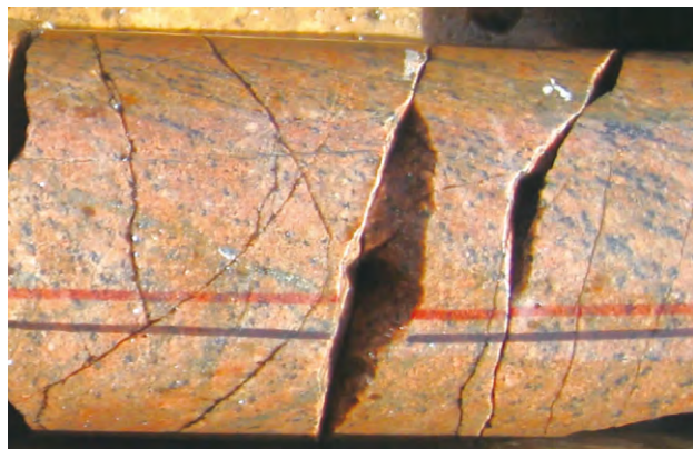
图10 标本中的磁铁矿特征
