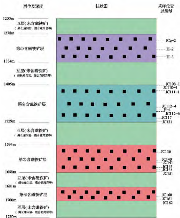
图9 JCSD(-1200~-1750m)钻孔柱状示意图
